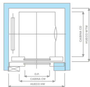
Croquis de planta un embarque puerta ap. central
