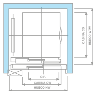
Croquis de planta un embarque puerta telescópica
